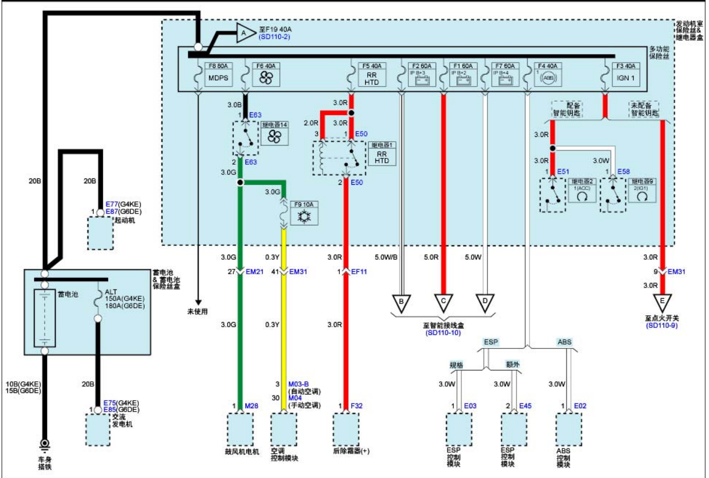
电源分布 (1)
